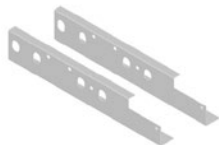
MC Befestigungssatz 3.6 Reserverad für Verlegung des AL-KO-Reserveradträgers um 90 mm nach hinten. 2 Stück Herst.-Nr.: 227-1145 Art-Nr. 115/093
