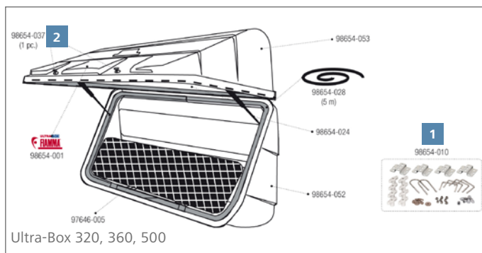
Befestigungs-Kit für Ultra-Box 1 Stück 98654-010 Art-Nr. 136/373
