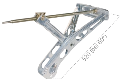
Steckstützen Premium Tragfähigkeit: 1250 kg; zul. Gewicht: 2500 kg; Gewicht: 5 kg Herst.-Nr.: 1224510 Art-Nr. 120/007
