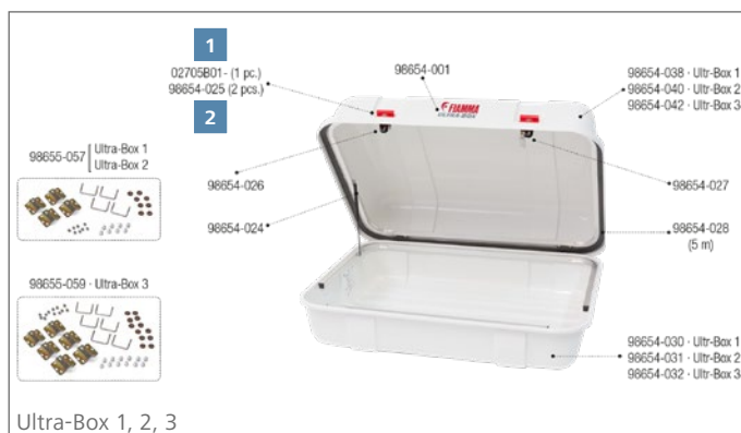
Handgriff mit Schloss 1 Stück 02705B01- Art-Nr. 136/615
