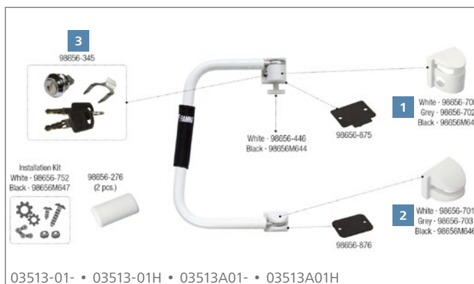
Abdeckung Security oben 1 Stück 98656-700 Art-Nr. 214/102
