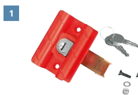
Handgriff mit Schloss 1 Stück 02705B01- Art-Nr. 136/615
