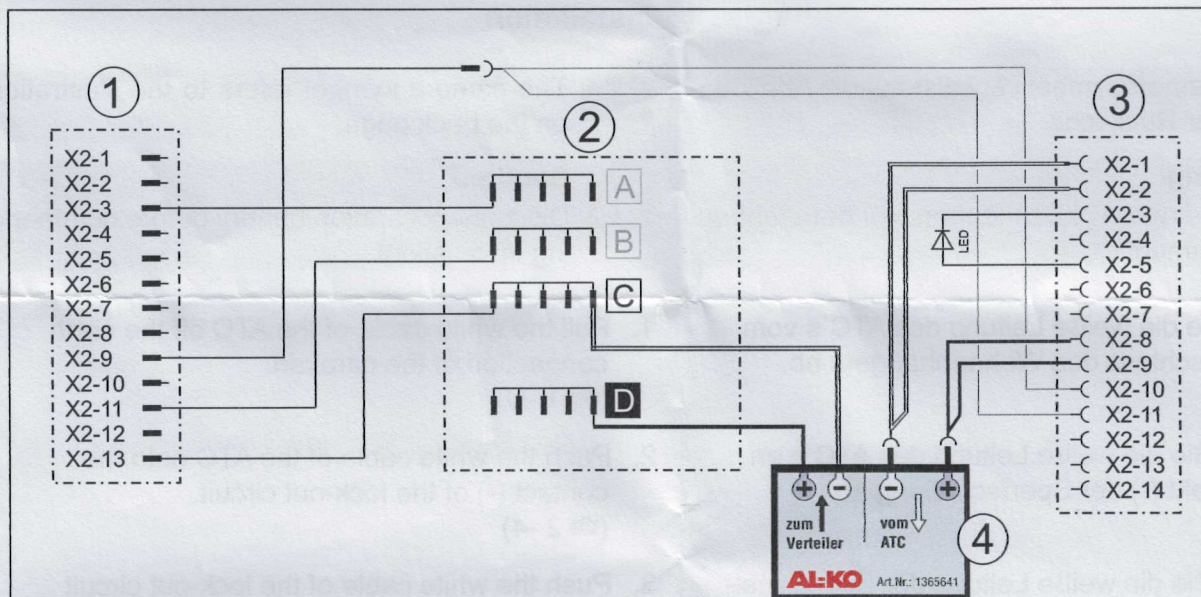
2 mit Sperrschaltung | with lock-out circuit
