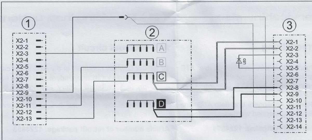
1 ohne Sperrschaltung | without lock-out circuit
