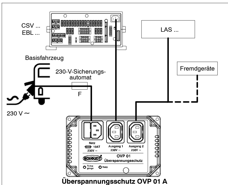
Bild 2 Prinzipielle Funktion des Überspannungsschutzes OVP 01 A
