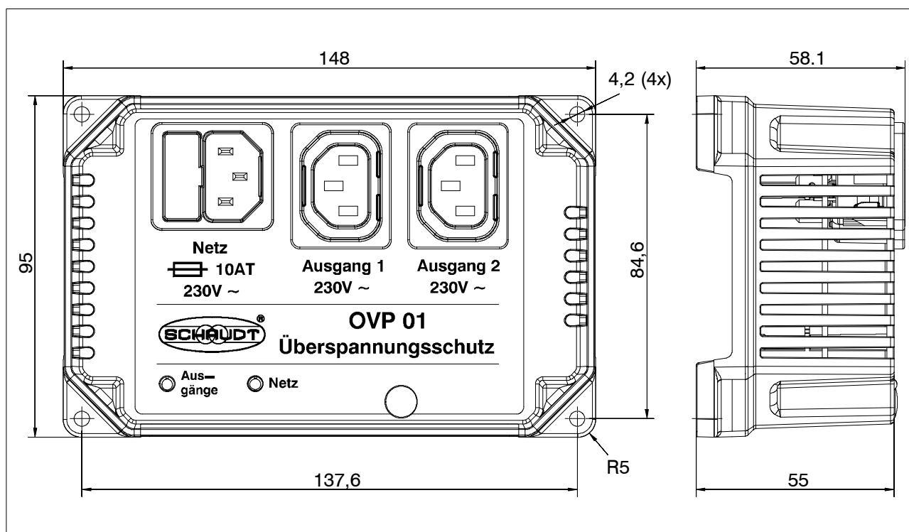
Bild 3 Maßbild Überspannungsschutz
