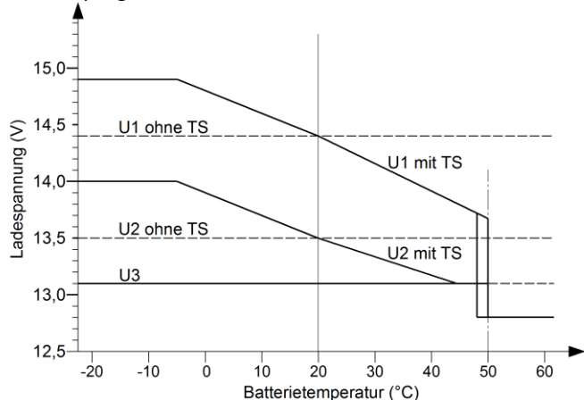
Ladeprogramm Säure „Lead Acid/AGM 1“, IU1oU2oU3
