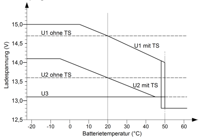
Ladeprogramm „AGM 2“, IU1oU2oU3
